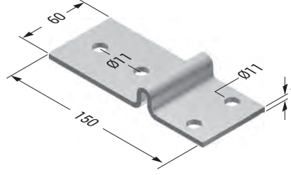
IDK Ek Elemanı
