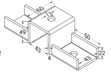
82x41 Çapraz Bağlantı Elemanı - Çift Yön
