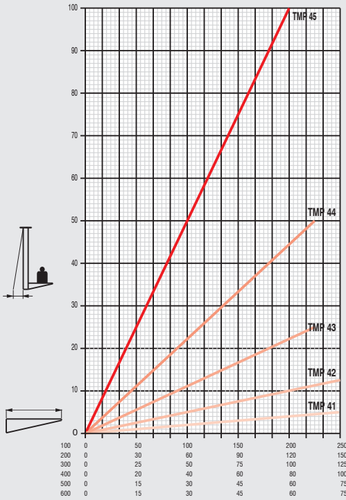
TMP 41-42-43-44-45 Maks. Yük ve Sehim Değerleri
